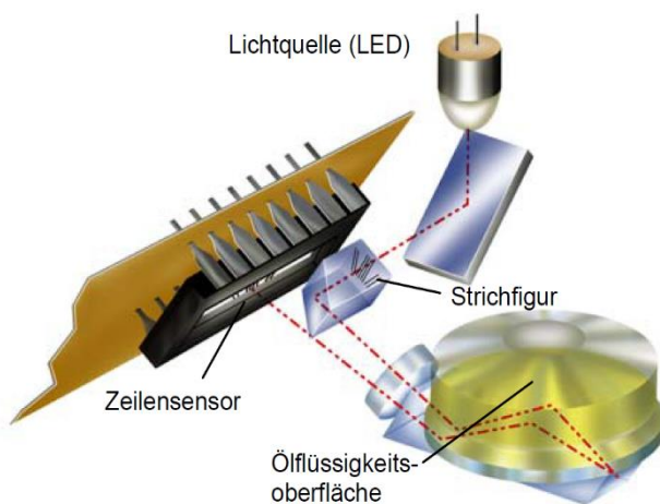
Abb. 5: Prinzip des digitalen Neigungssensors 99 (@ Leica Geosystems).
