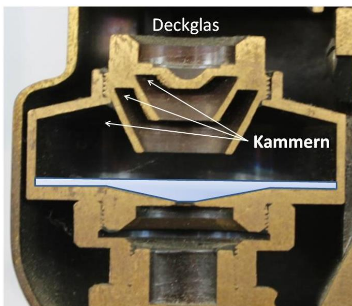
Abb.1: WILD T1A Kompensator (@ Leica Geosystems).
