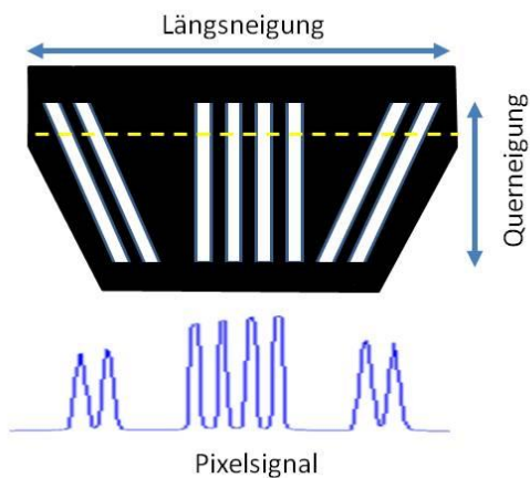
Abb. 4: Strichfigur und digitales Signal (@ Leica Geosystems).
