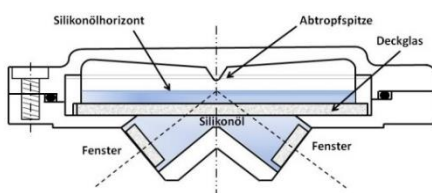
Abb. 3: Der T2000 Flüssigkeitshorizont (@ Leica Geosystems).
