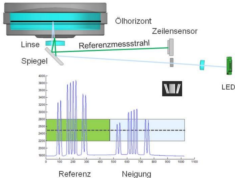
Abb. 6: Prinzip des "Belo Horizonte" Neigungssensors (@Leica Geosystems).
